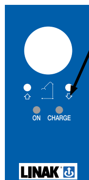
Elektrisk nödsänkning
